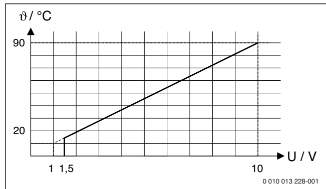
sl. 65 Linearna zavisnost između signala od 0-10 V (napon u voltima) i potrebne temperature polaznog voda \theta (u °C u odnosu na opseg od minimalne temperature polaznog voda do maksimalne temperature polaznog voda [osnovno podešavanje 20 °C do 90 °C])
