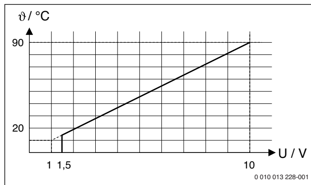
Fig. 44 Combi-nația liniară dintre semnalul 0-10V (U în volți) și temperatura solicitată a turului \Theta (în °C bazată pe domeniul de temperatură minimă a turului până la temperatura maximă a turului [setare din fabrică 20 °C până la 90 °C])
