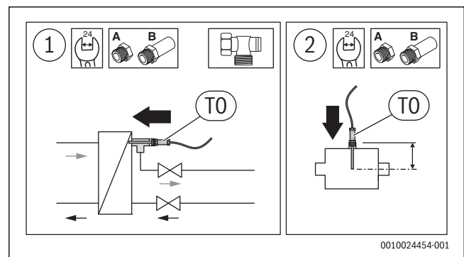
Pav. 31 Optimizuotas jutiklio montavimas
