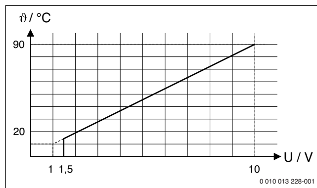
Sl.58 Linearna zveza med signalom 0–10 V (U v Voltih) in zahtevano temperaturo dvižnega voda \vartheta (v °C glede na območje od minimalne do maksimalne temperature dvižnega voda [osnovna nastavitev 20 °C do 90 °C])
