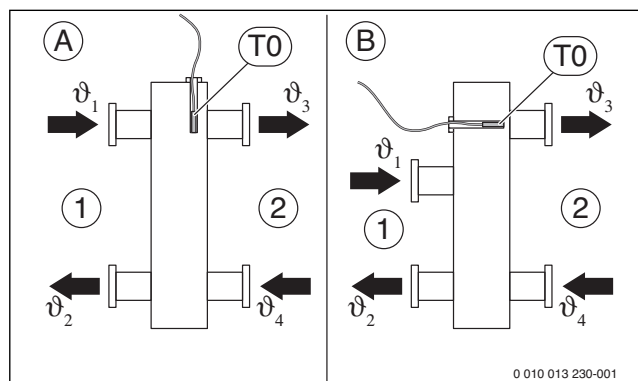
Фиг. 5 Позиция температурен датчик в линията на подаването (T0)
