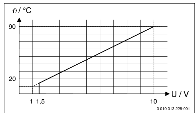
Joon. 9 Lineaarne sõltuvus 0–10 V signaali (U, voltides) ja vajaliku pealevoolutemperatuuri vahel \theta (°C vahemikus minimaalsest pealevoolutemperatuurist kuni maksimaalse pealevoolutemperatuurini [põhiseadistus 20 °C kuni 90 °C])
