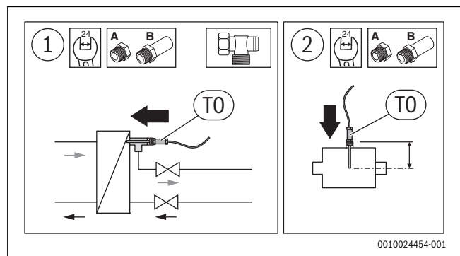
sl. 66 Optimizovana montaža senzora
