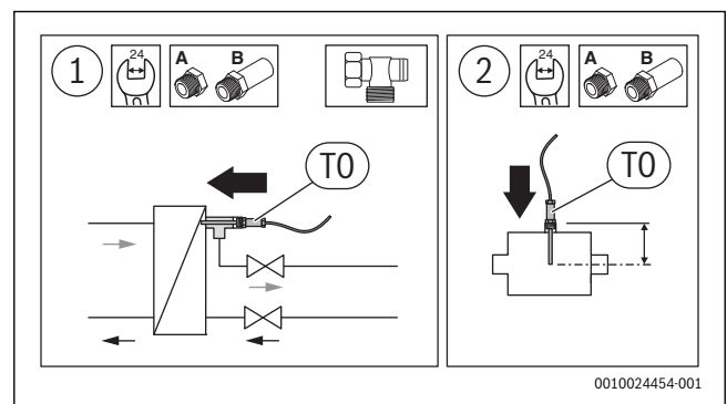
Рис. 52 Оптимальный монтаж датчика
