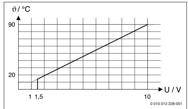
Att. 37 Lineāra saistība starp 0-10V signālu (U voltos) un pieprasītās turpgaitas temperatūras \theta (°C attiecībā uz minimālās līdz maksimālās turpgaitas temperatūras diapazonu [pamatīestātijums 20 °C līdz 90 °C])
