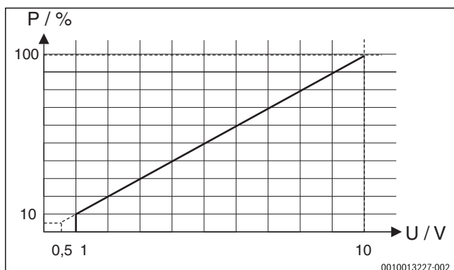
Att. 36 Lineārā attiecība starp 0-10 V signālu (U voltos) un pieprasīto jaudu P (procentos attiecībā uz sistēmas maksimālo jaudu)
