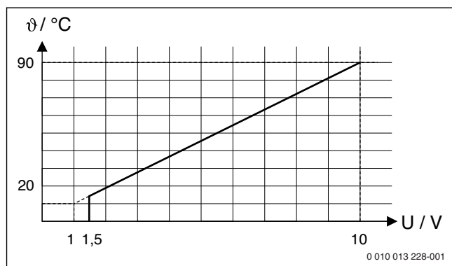
Фиг. 2 Линейна зависимост между сигнала 0 – 10 V ( U във волтове) и изискваната температура на подаване \vartheta (в °C по отношение на обхвата минимална температура до максимална температура на подаване [основна настройка 20 °C до 90 °C])
