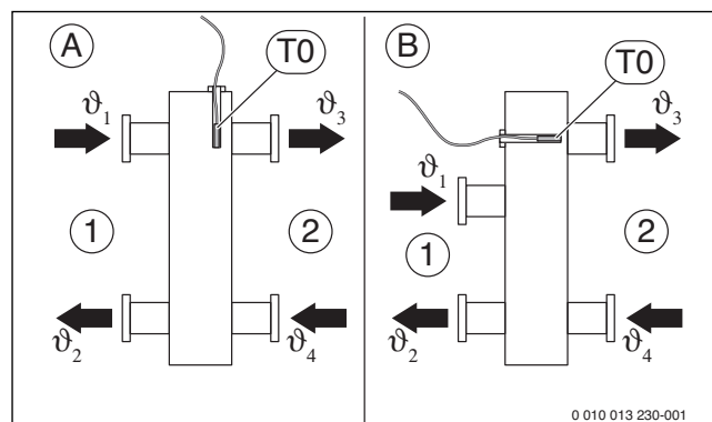
26. ábra Hőmérséklet érzékelő az előremenő ágban (T0)
