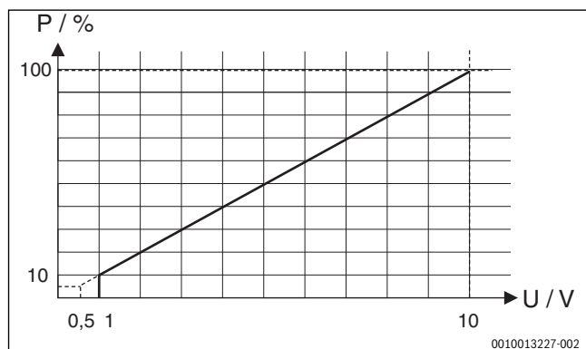
sl. 64 Linearna zavisnost između signala od 0-10 V (napon u voltima) i potrebne snage P (procenat u odnosu na maksimalnu snagu sistema)
