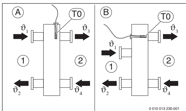
Fig. 47 Poziție senzor de temperatură de tur (T0)
