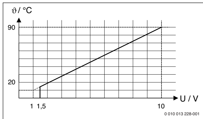
Рис. 51 Линейная зависимость между сигналом 0-10В и требуемой температурой подающей линии \vartheta (в °C относительно диапазона от минимальной до максимальной температуры подающей линии [первоначальное значение 20 °C - 90 °C])
