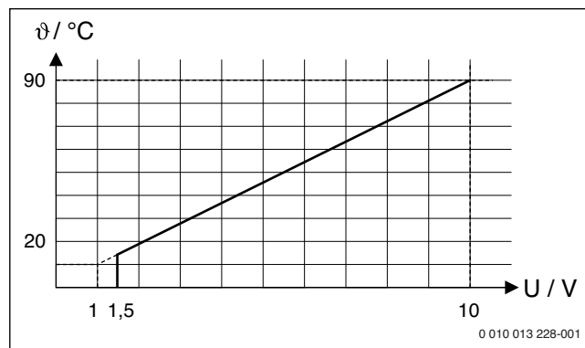
Sl. 16 Linearni odnos između signala 0-10 V ( U u volt) i zatražene temperature polaznog voda \vartheta ( u °C postocima naspram područja minimalne do maksimalne temperature polaznog voda [osnovna postavka 20 °C do 90 °C])
