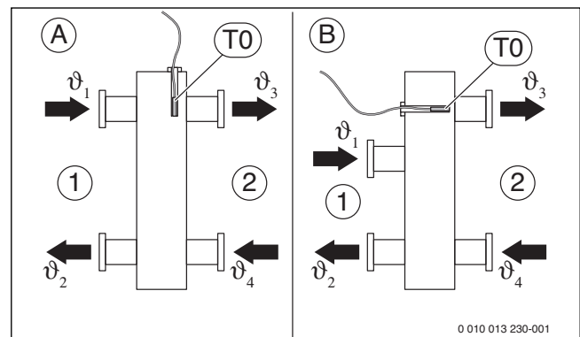
Pav. 33 Tiekiamo srauto temperatūros jutiklio padėtis (T0)
