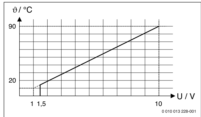
Pav. 30 Tiesinis ryšys tarp 0-10V signalo (U, voltais) ir reikalaujamos tiekiamo srauto temperatūros \theta ( ^{\circ}\text{C} diapazono nuo minimalios tiekiamo srauto temperatūros iki maksimalios tiekiamo srauto temperatūros atžvilgiu [gamyklinis nustatymas nuo 20^{\circ}\text{C} iki 90^{\circ}\text{C} ])
