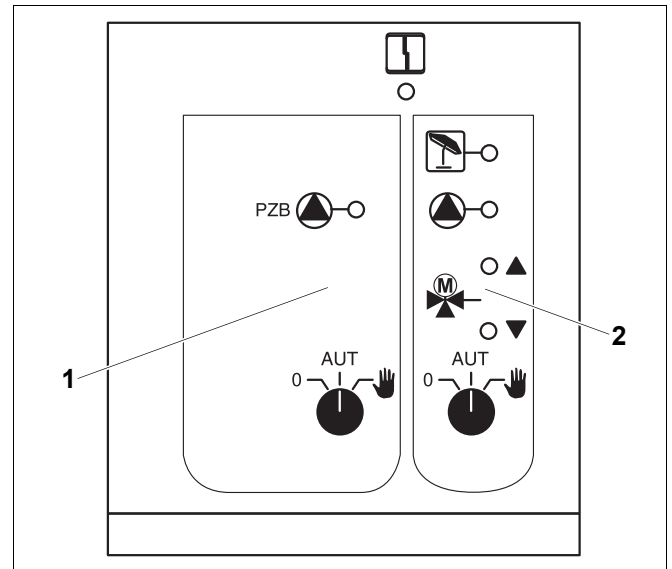
Рис. 21 Центральный модуль ZM433
