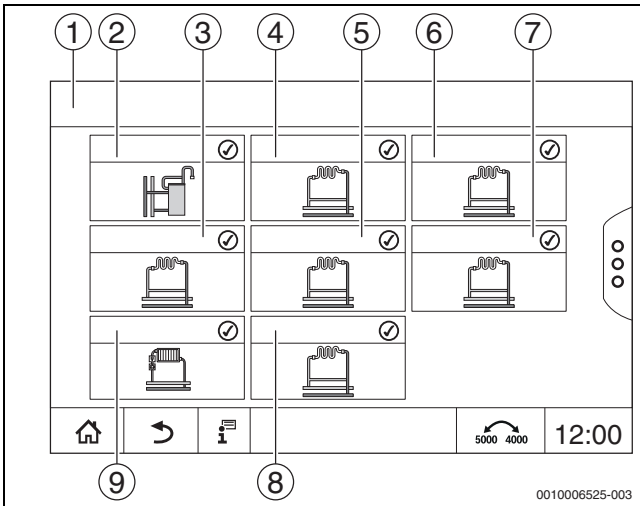
Рис. 9 Обзор отопительных контуров (пример)
