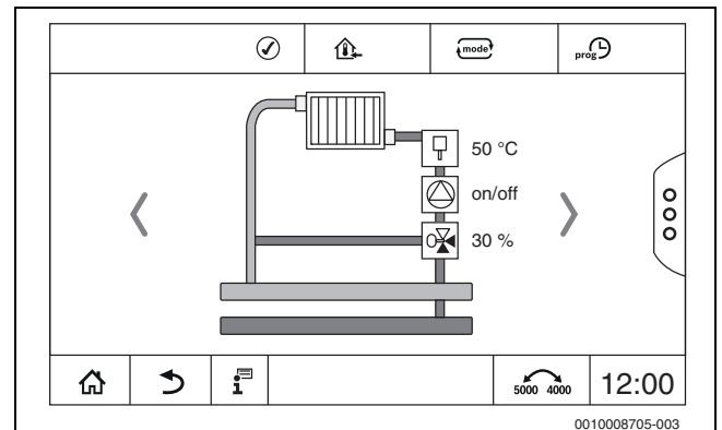
Рис. 13 Обзор отопительного контура серии 5000
