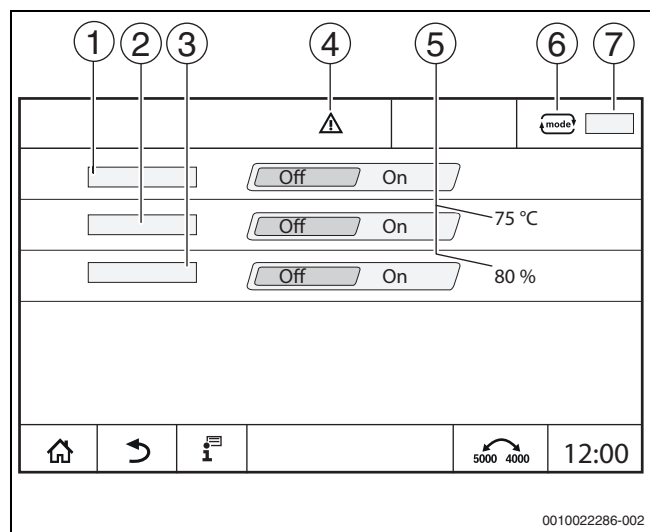
Рис. 18 Индикация Ручной режим
