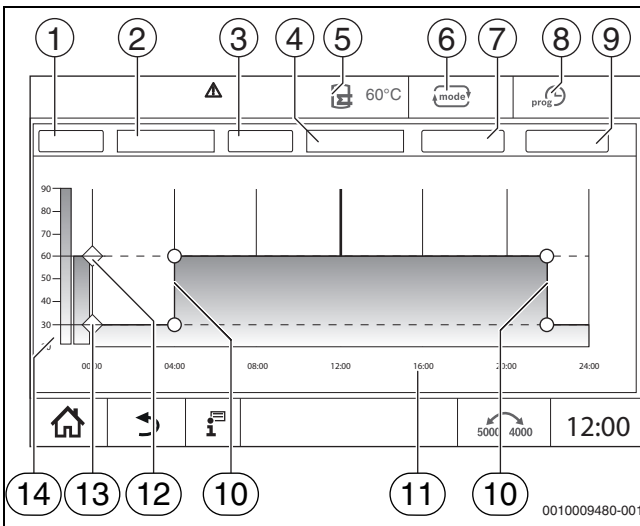
Рис. 29 Программа приготовления горячей воды
