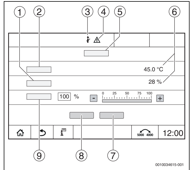
Рис. 17 Индикация Тест дымовых газов > настройки котла
