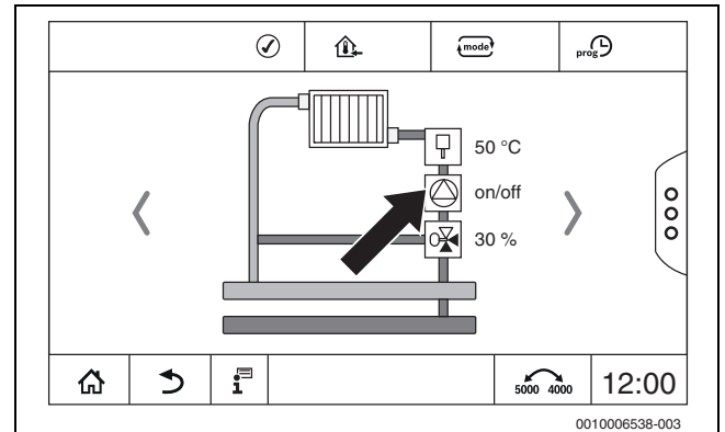
Рис. 12 Выбор компонента установки
