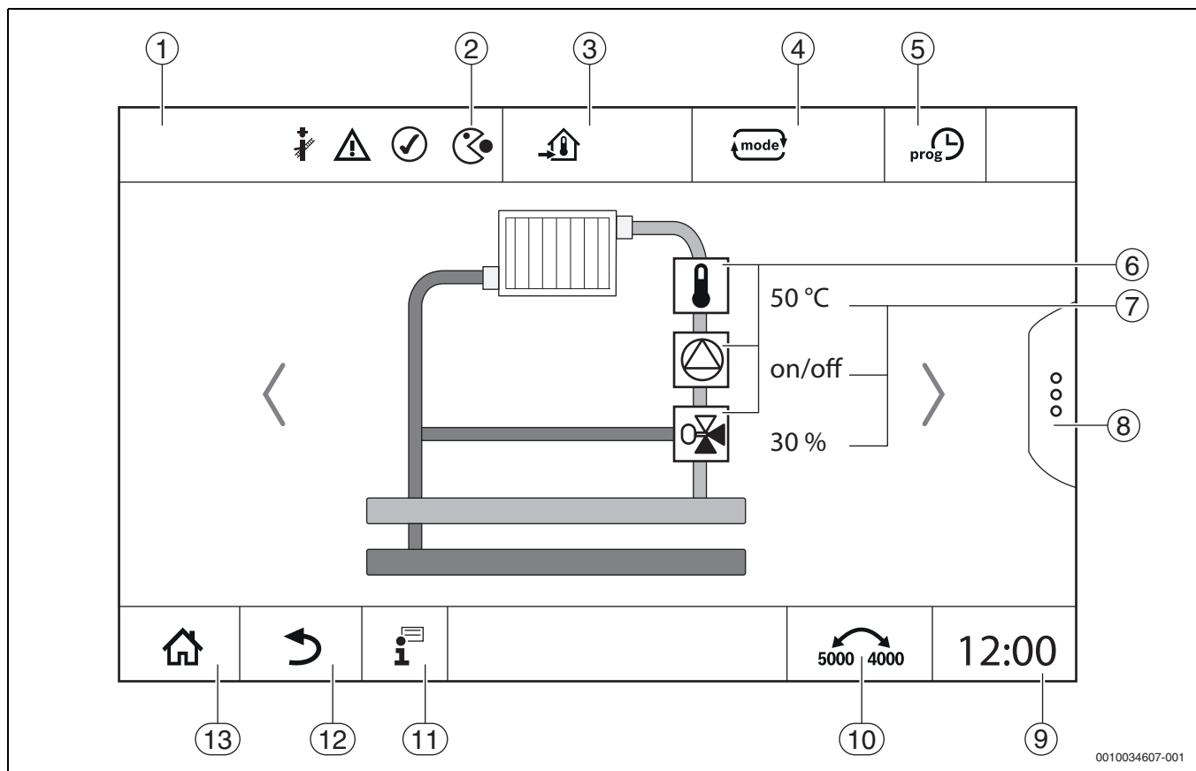
Рис. 7 Элементы управления и индикации (пример)
