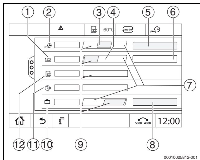
Рис. 25 Дополнительные функции контуров ГВС
